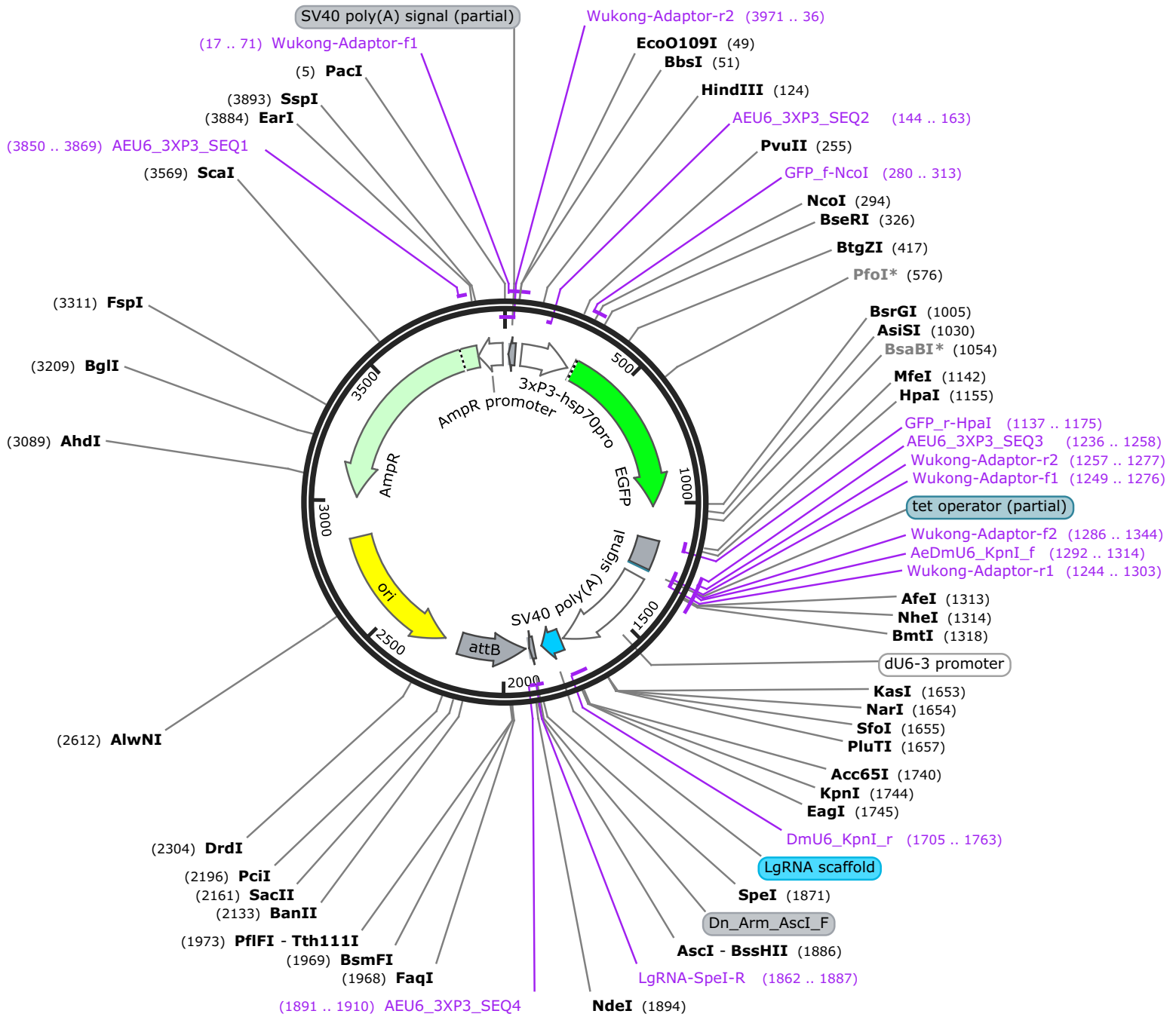
1596_pDmU6-LgRNA-3xp3-GFP 3990 bp
